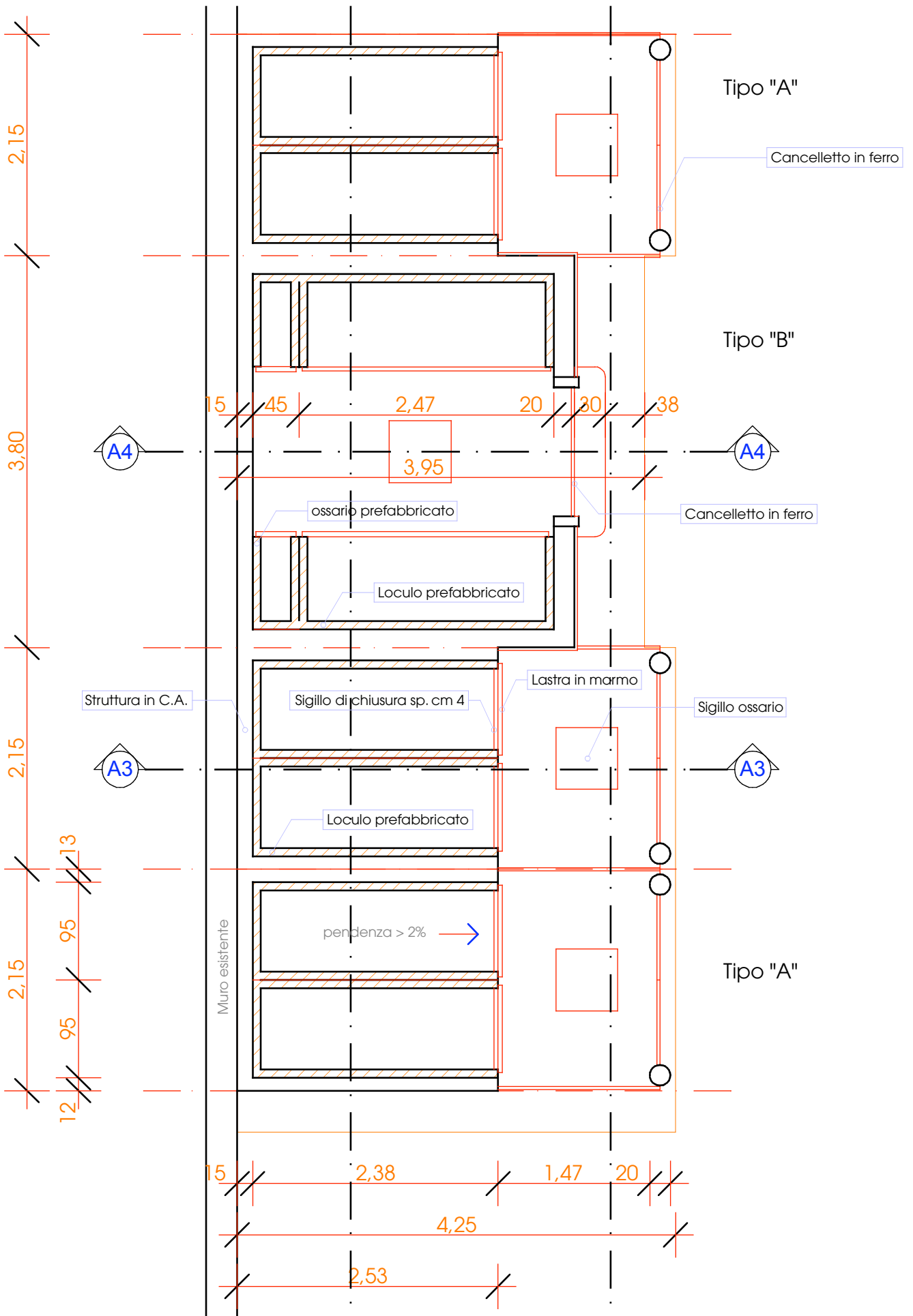
Allegato 2.1 - Pianta tombe tipo "A" e "B" - scala 1:50
