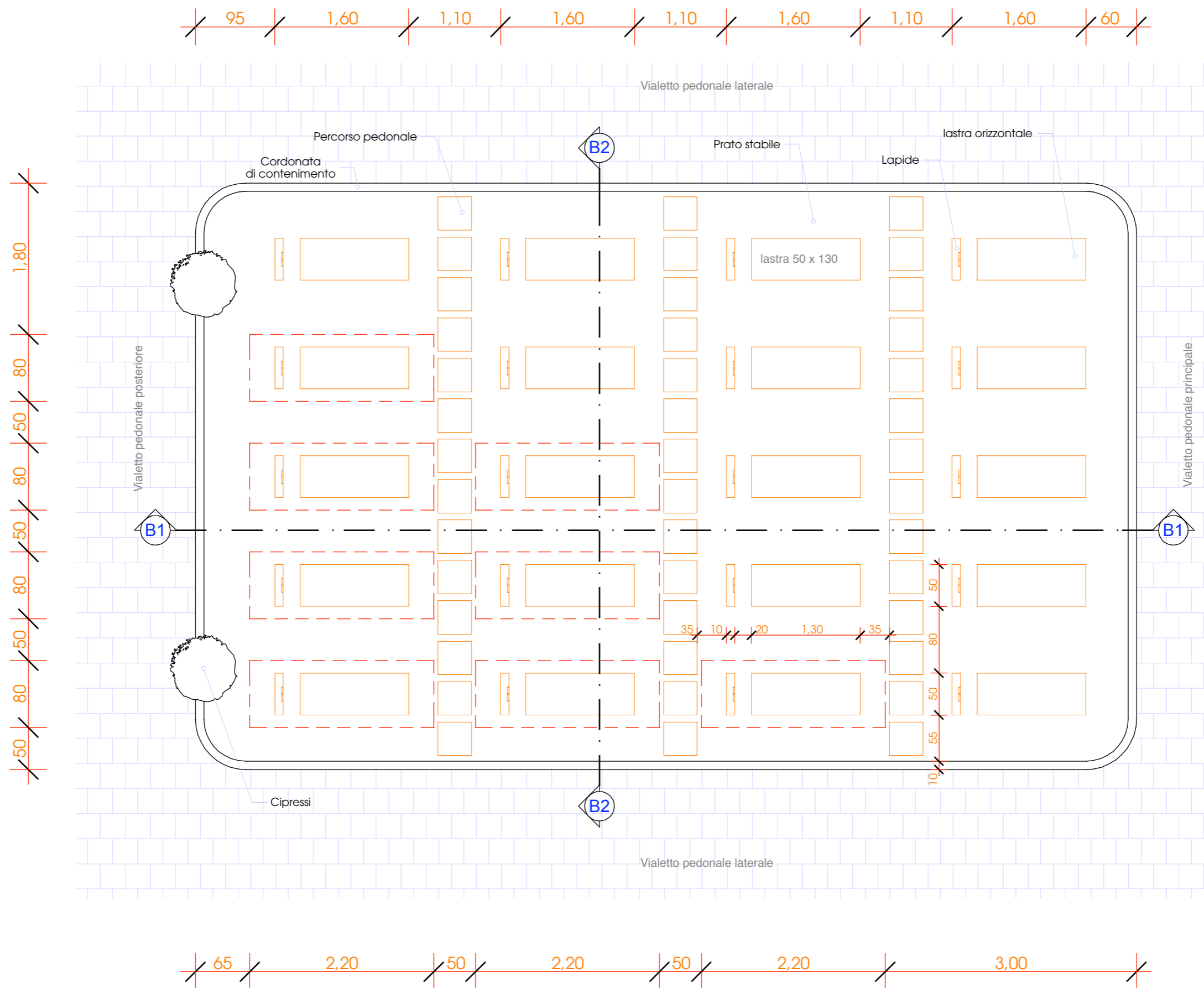
Allegato 3.1 - Pianta campo tipo per inumazione - scala 1:50
