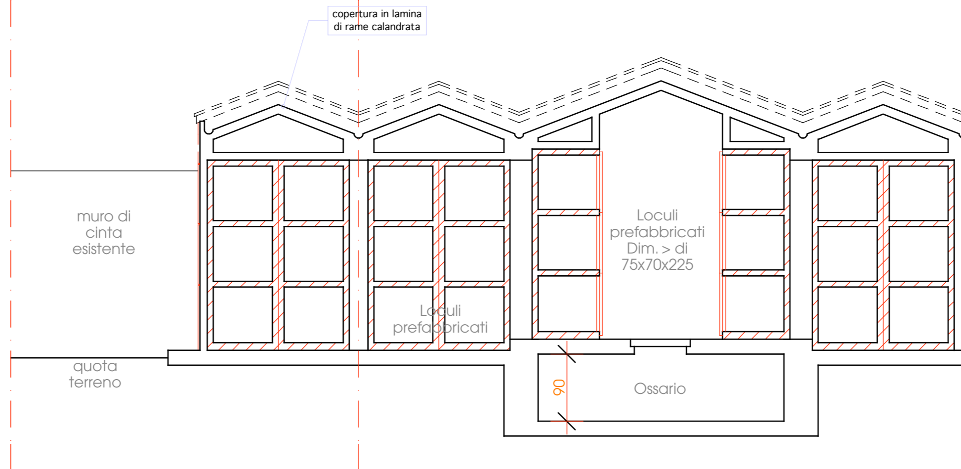
Sezione A1
